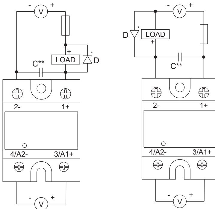
Fig. 9 RM1D-Anschlusschaltpläne
