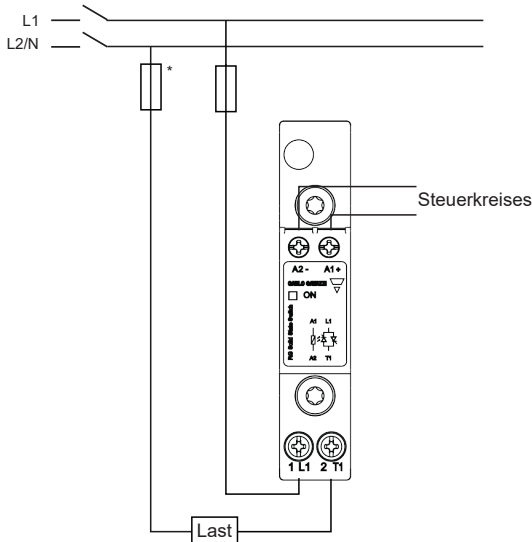
Variante ohne Übertemperaturüberwachung
