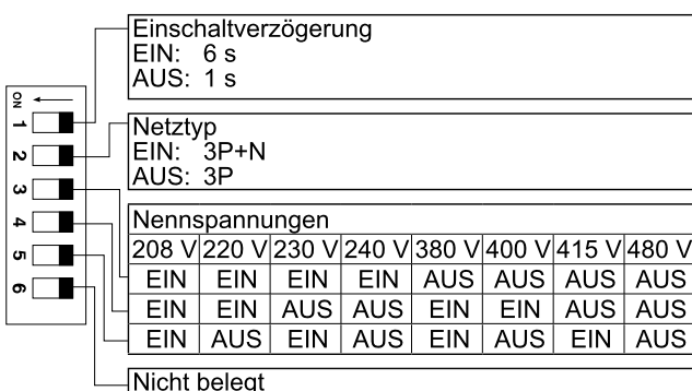
Abb. 1 Tabelle der DIP-Schalter-Einstellungen M44
