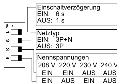
Abb. 2 Tabelle der DIP-Schalter-Einstellungen M23
