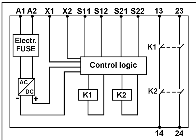
Fig. 2 - Schema circuitale dei moduli NSC02D / NSC02D circuit diagram
