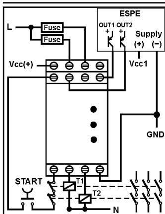
Fig. 3: ESPE: 2 uscite PNP a 1 filo / Two 1-wire PNP outputs
