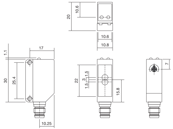
LD30CNB...M5IO
