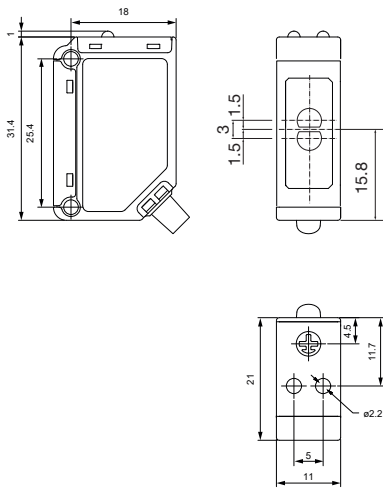
LD30ETB...A2IO
