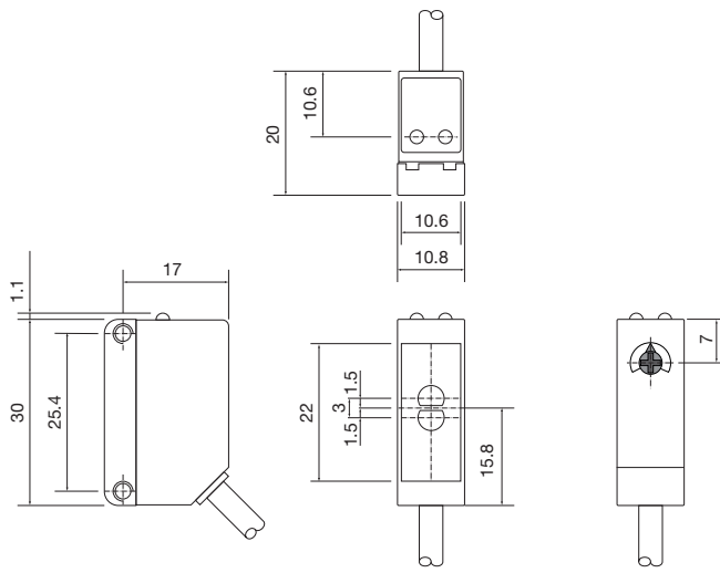
LD30CNB...A2IO
