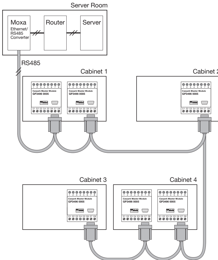
Fig. 62: Extended wiring
