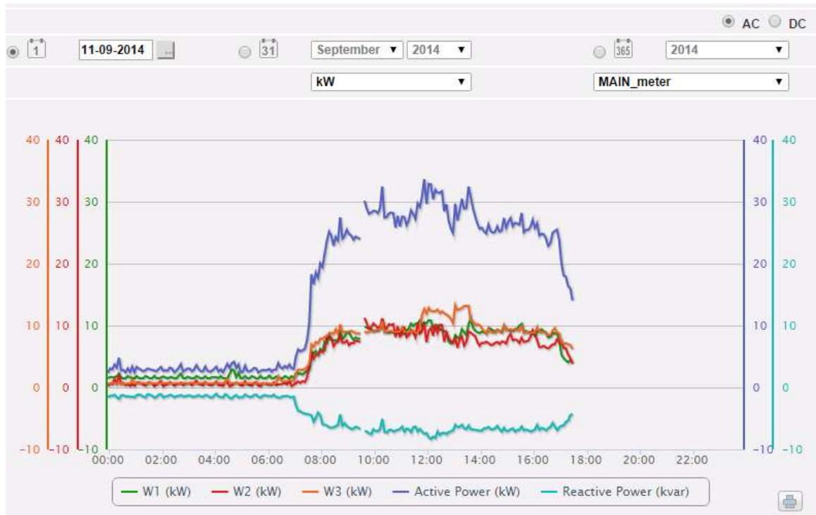
Grafico andamento potenze di sistema (kW e kvar)
