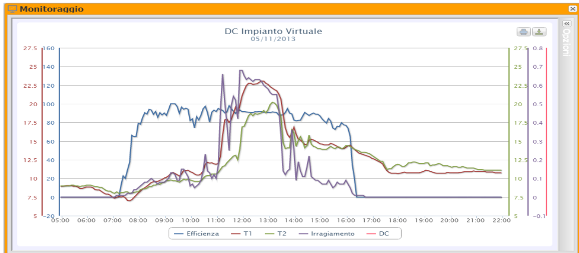
Figure 12: Finestra Monitor; Grafico Potenza CC.
