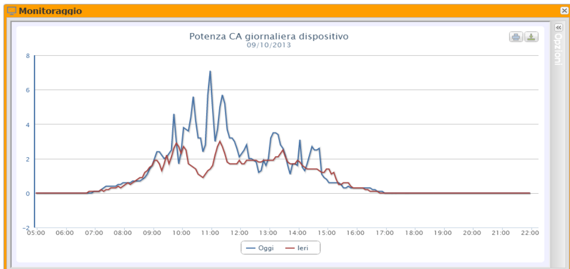
Figure 8: Finestra Monitor – Grafico Produzione AC
