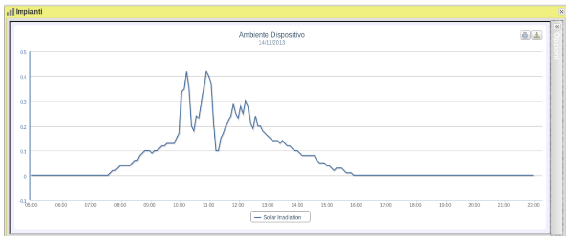
Figure 40: Finestra Impianto, Grafico Sensori “Irraggiamento”.
