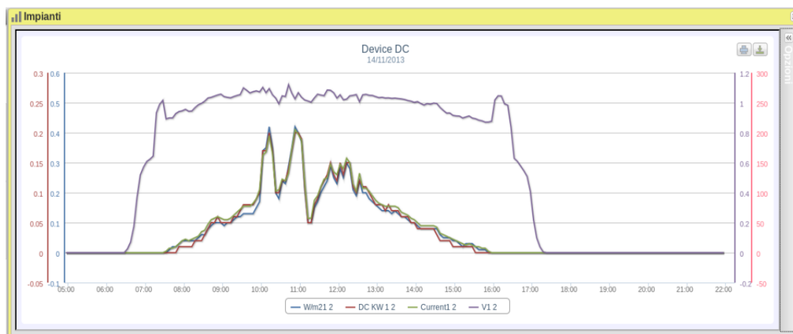
Figure 30: Finestra Impianto, Grafico Produzione DC “Singola Stringa – KW+A+V+W/m2”.
