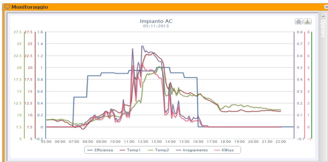
Figure 16: Finestra Monitor; Grafico Potenza CA.
