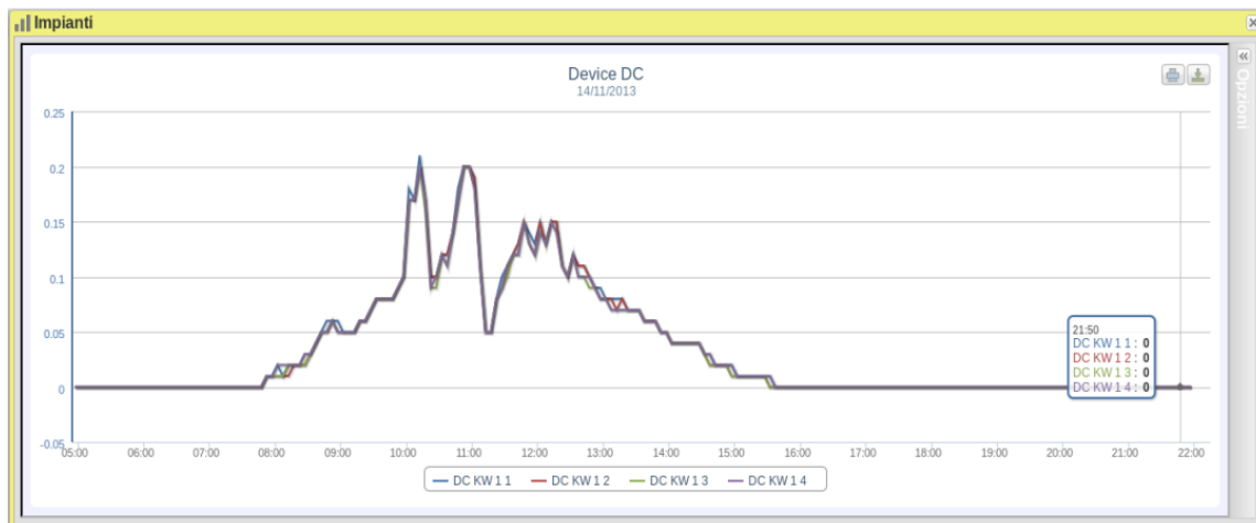
Figure 29: Finestra Impianti; Grafico Produzione DC – Selezione “Singola Stringa”.
