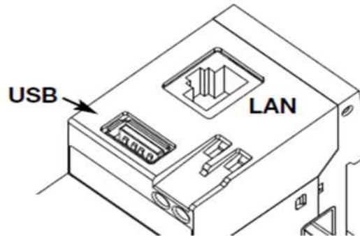
Port USB pour clé USB
