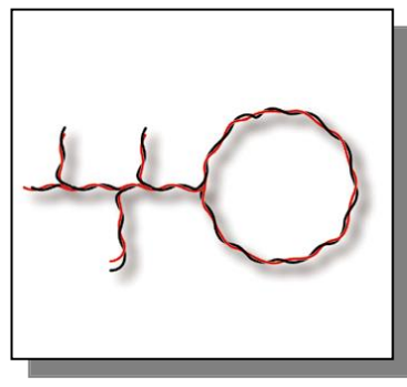
Combinada: la mejor ubicación para SH2MCG24 es el centro, entre los dos módulos más alejados.
