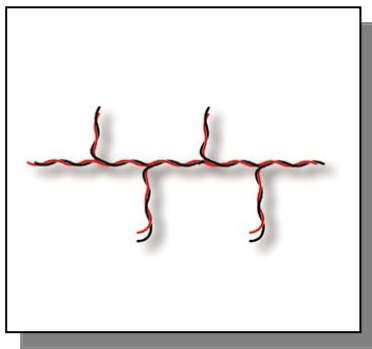
En línea recta: el mejor lugar para el SH2MCG24 es el centro de la línea
