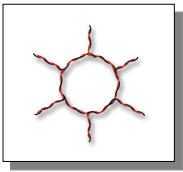
En anillo: la mejor ubicación para el SH2MCG24 es el centro, entre los dos módulos más alejados.
