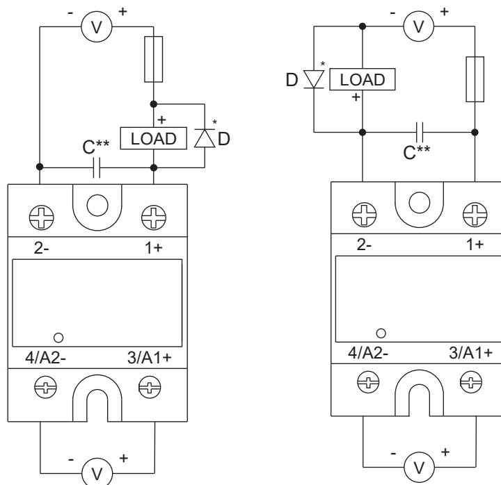
Fig. 9 Diagramas de conexión de la serie RM1D
