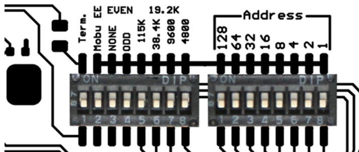
Fig. 10: Dettaglio DIP switch
