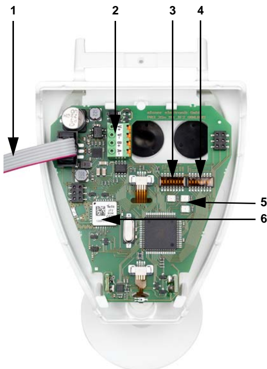
Fig. 9: Riepilogo scheda
