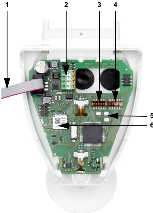
Fig. 8: Vista general placa de circuito impreso (PCB)
