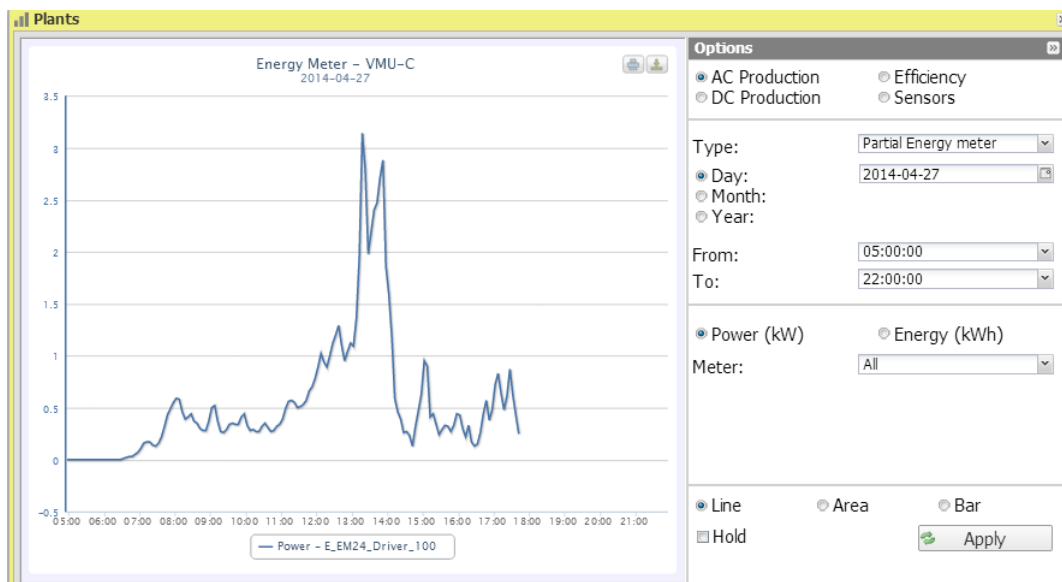
Figura 23: Ventana de la planta; Gráfico del contador de energía– Selección de opción del contador de energía parcial.
