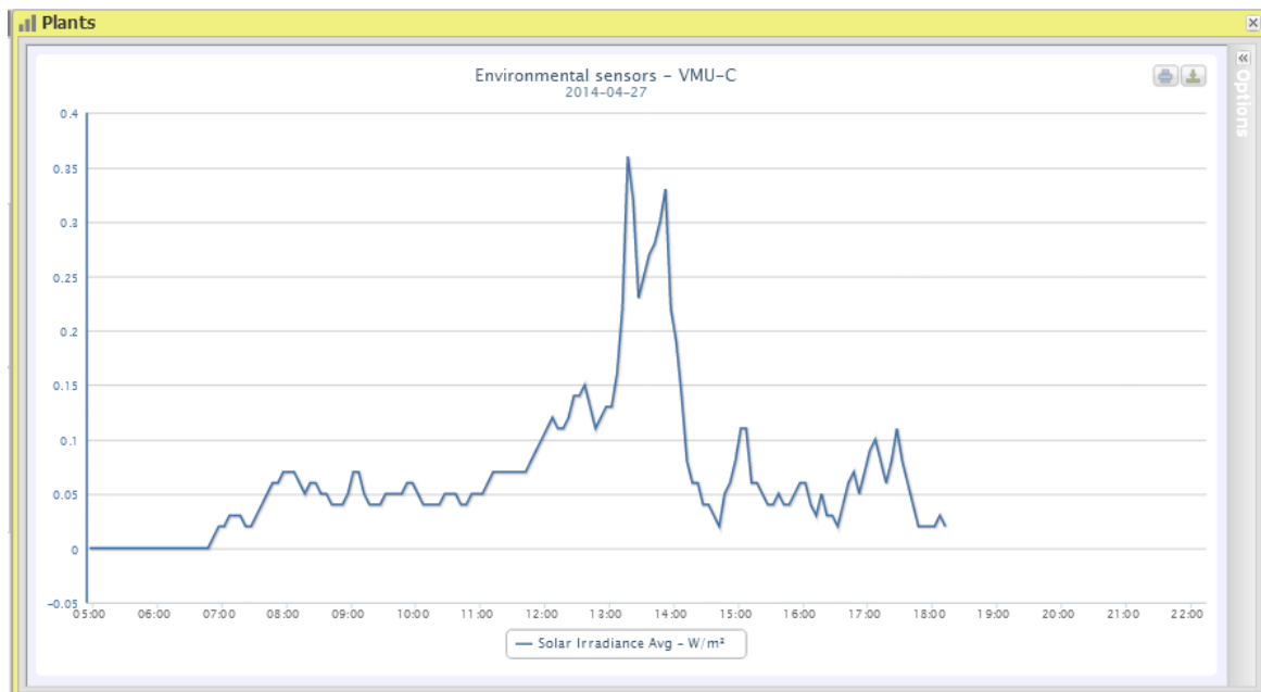
Figura 39: Ventana de la planta; Gráfico del sensor "Radiación".
