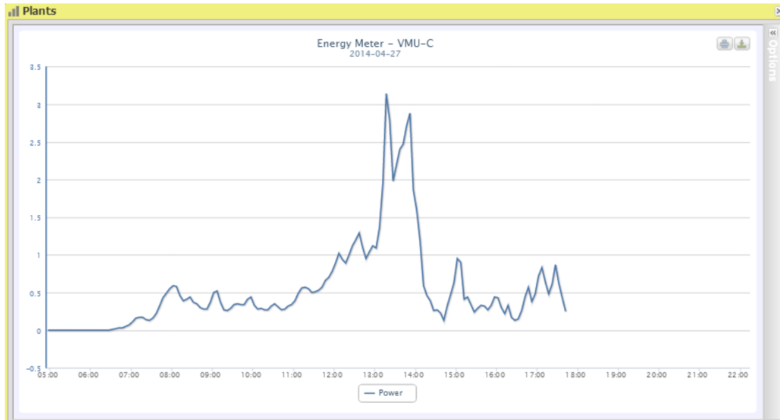
Figura 21: Ventana de la planta; Gráfico del contador de energía– Selección de opción del contador de energía total.
