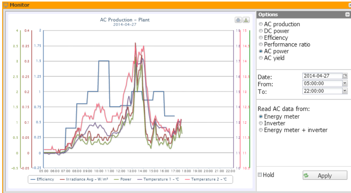
Figura 15: Ventana del monitor; Gráfico de alimentación de CA.
