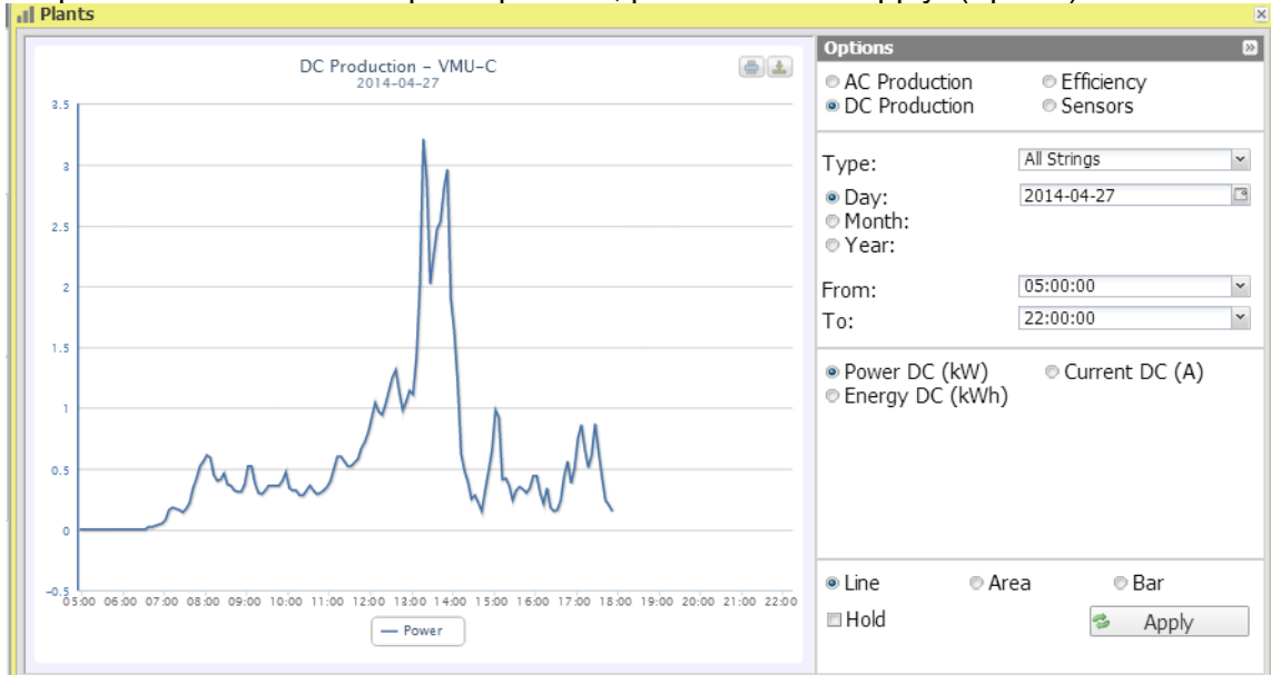
Figura 25: Ventana de la planta; Gráfico de producción de CC – Selección de opción de “Todas las cadenas”
