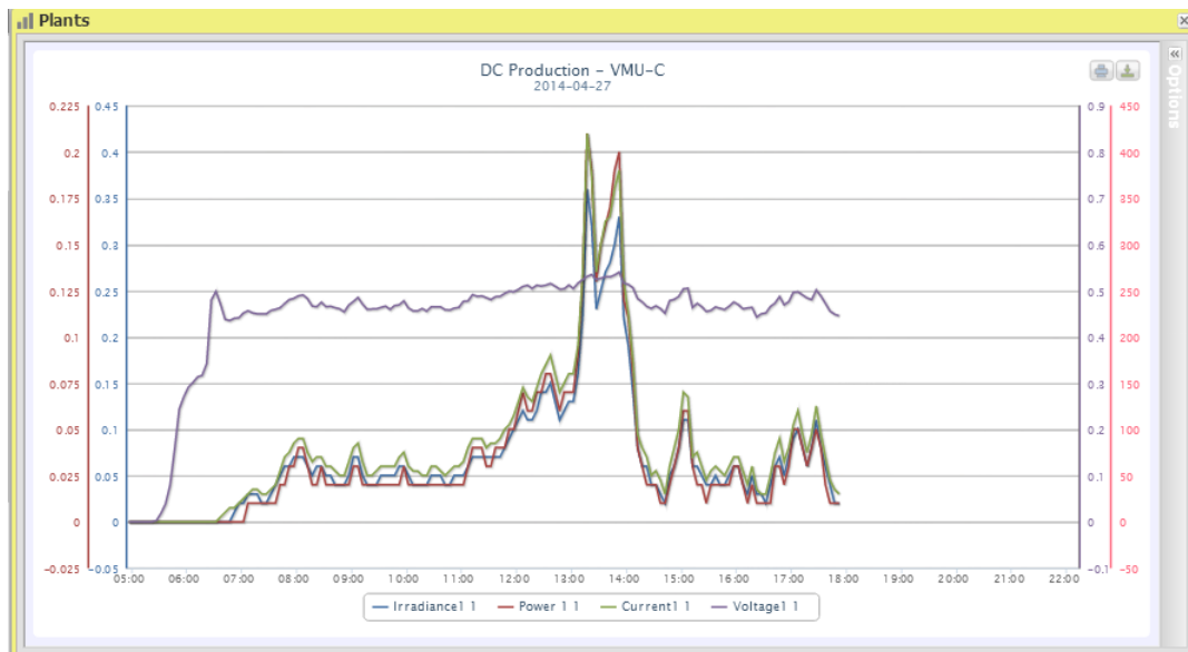
Figura 29: Ventana de la planta, Gráfico de producción de CC “Cadena individual – KW+A+V+W/m2”.
