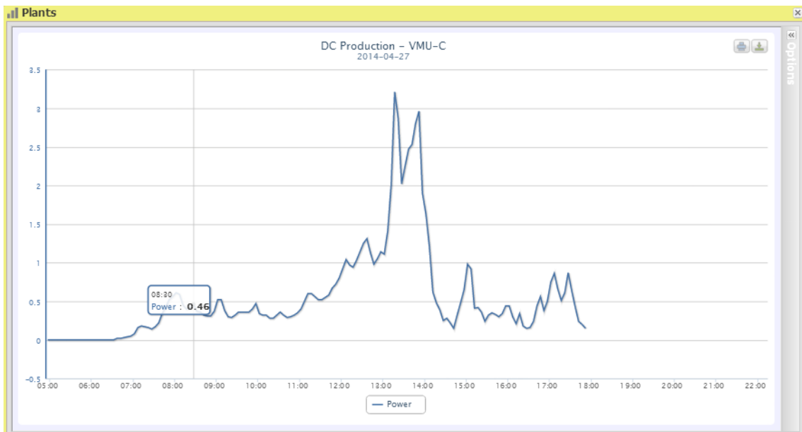
Figura 26: Ventana de la planta; Gráfico de producción de CC – Todas las cadenas
