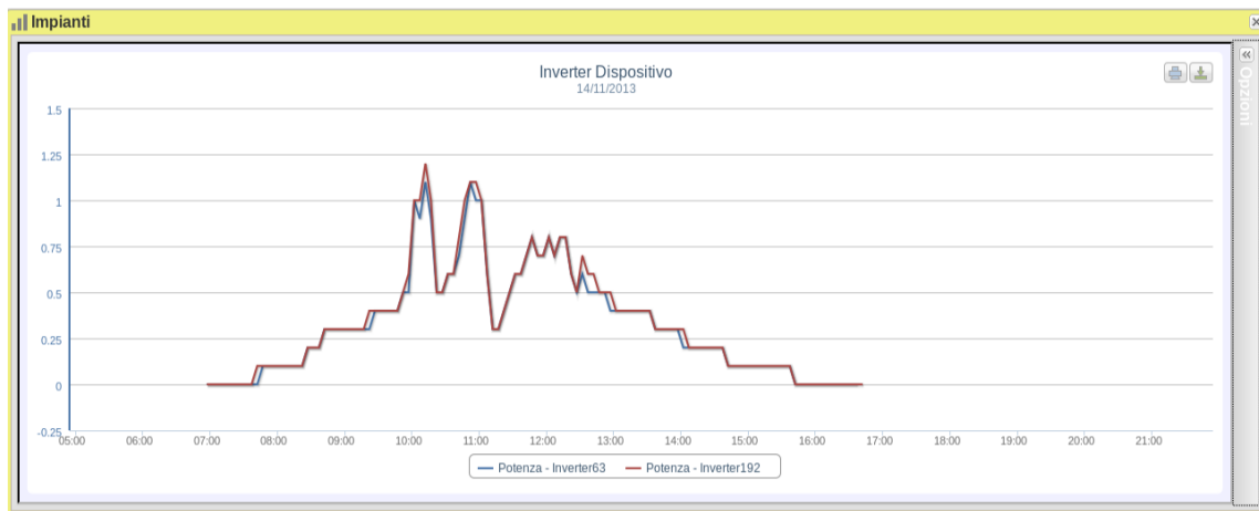
Figura 20: Ventana de la planta; Gráfico del inverter – Selección de opción de un inversor individual.
