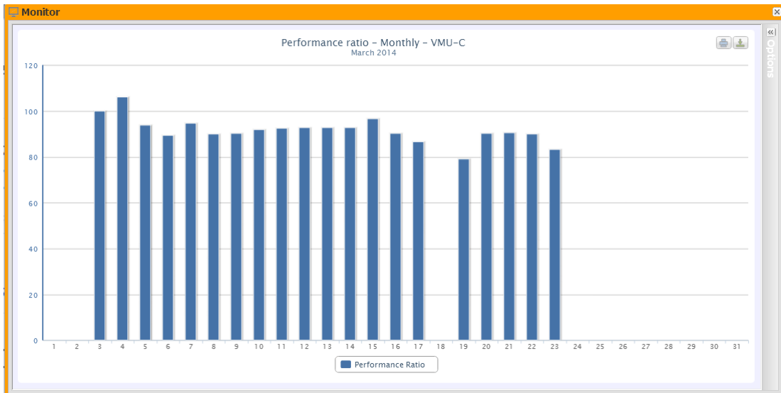
Figura 13: Ventana del monitor; Gráfico de rendimiento
