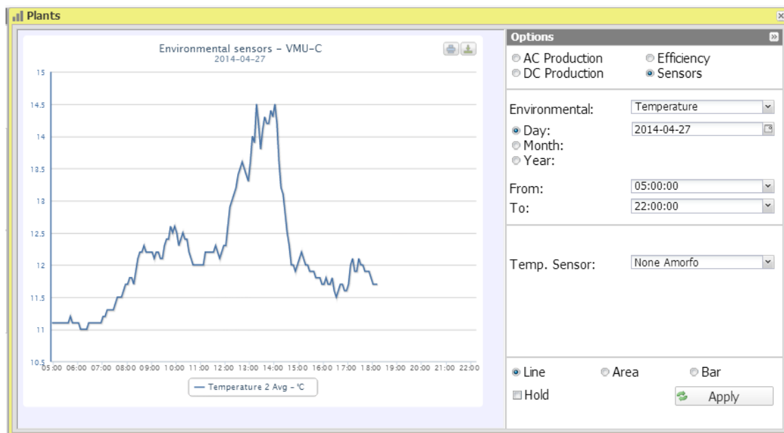
Figura 41: Ventana de la planta; Gráfico del sensor "Temperatura" - Opciones.
