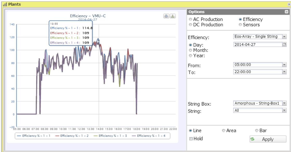
Figura 34: Ventana de la planta; Gráfico de eficiencia "Cadena individual" - Panel de opciones.
