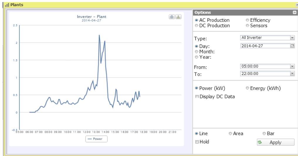
Figura 18: Ventana de la planta; Gráfico del inverter – Selección de opción
