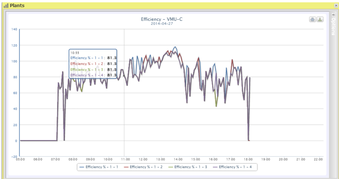
Figura 33: Ventana de la planta; Gráfico de eficiencia "Cadena individual".
