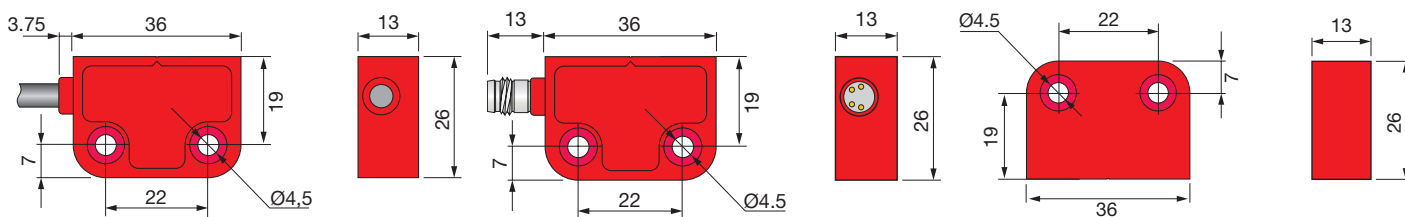
Fig. 1 - Dimensioner
