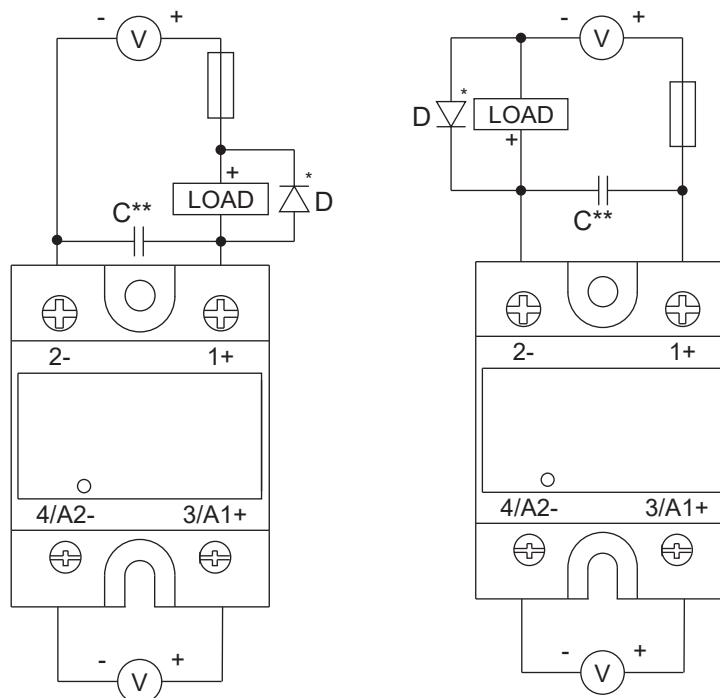
Fig. 9 RM1D-forbindelsesdiagrammer
