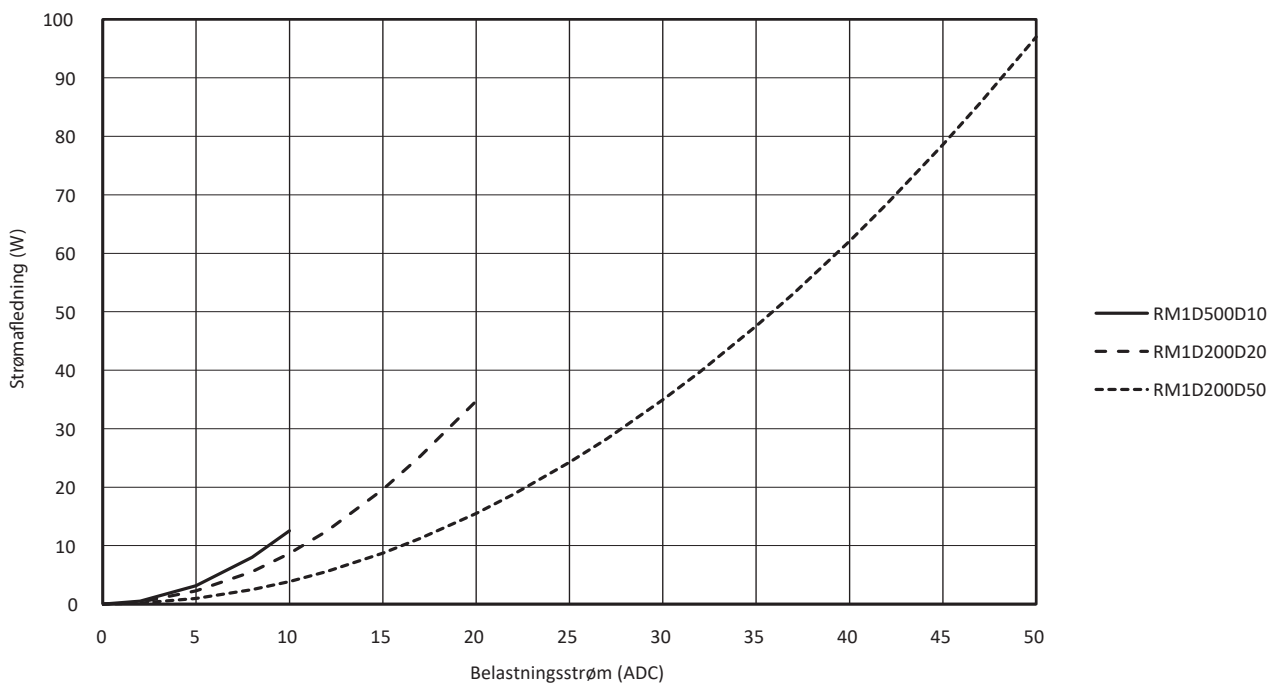
Fig. 8 Udgangsfordelingsgraf
