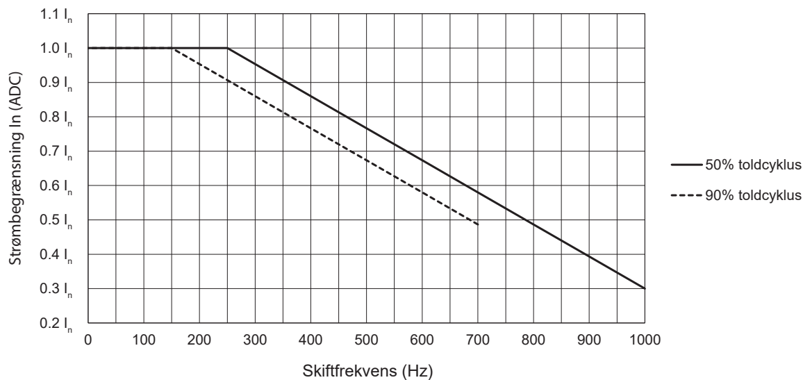
Fig. 6 Strømbegrænsning vs. skiftfrekvens 4
