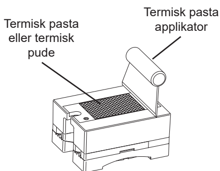
Fig. 11 Et fint lag termisk ledende siliciumpasta skal fordeles jævnt på SSR-basen, før montering på en køleplade. Alternativt kan man anvende en termisk plade. Materialet i den termiske interface påvirker den termiske ydelse. Sørg for, at kølepladen har den rette størrelse.
