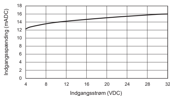
Fig. 3 Indgangsspænding vs. indgangsstrøm
