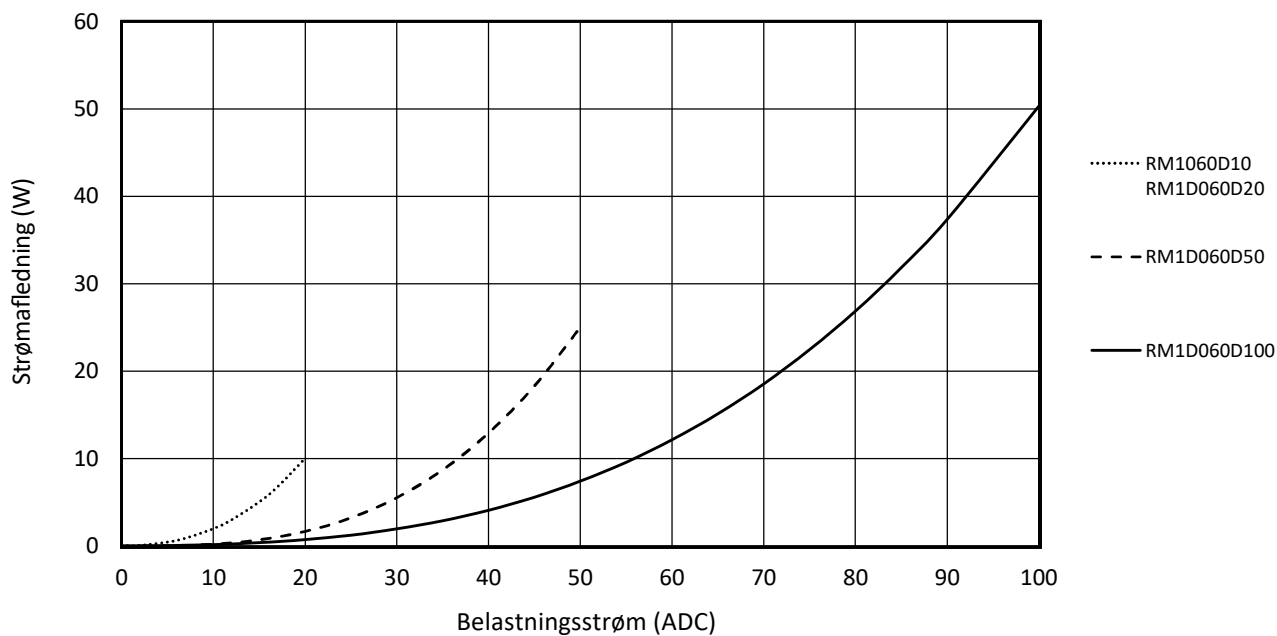
Fig. 7 Udgangsfordelingsgraf
