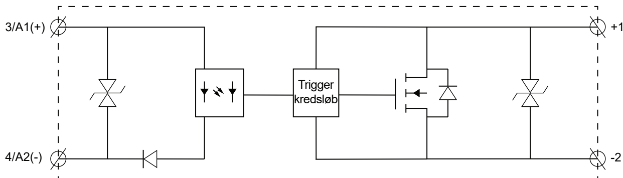
Fig. 10 RM1D funktionsdiagram
