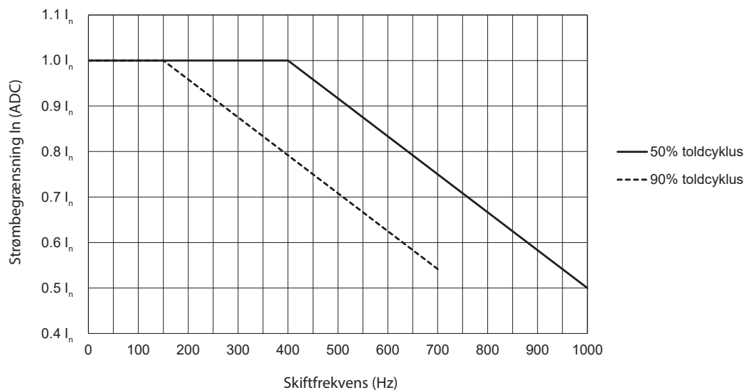
Fig. 5 Strømbegrænsning vs. skiffrekvens 4
