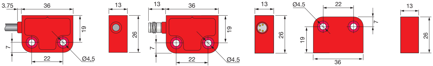
Abb. 1 - Abmessungen
