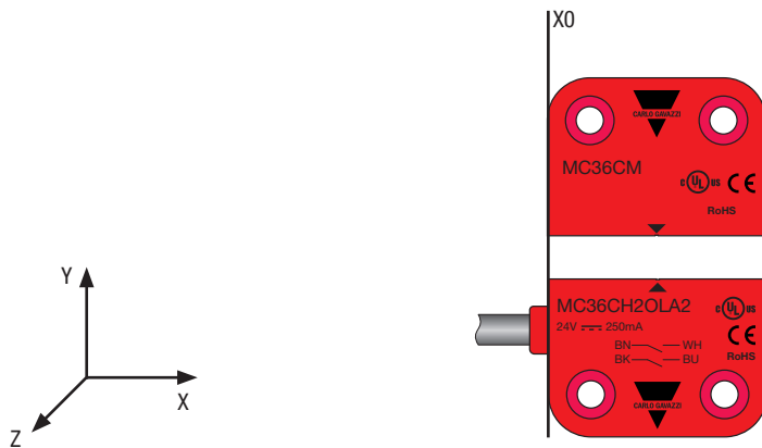
Abb. 2 - Betrieb und Ausrichtung der Sensoren
