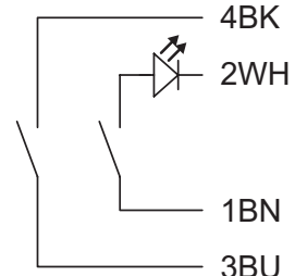
2NO, Kabel mit LED
