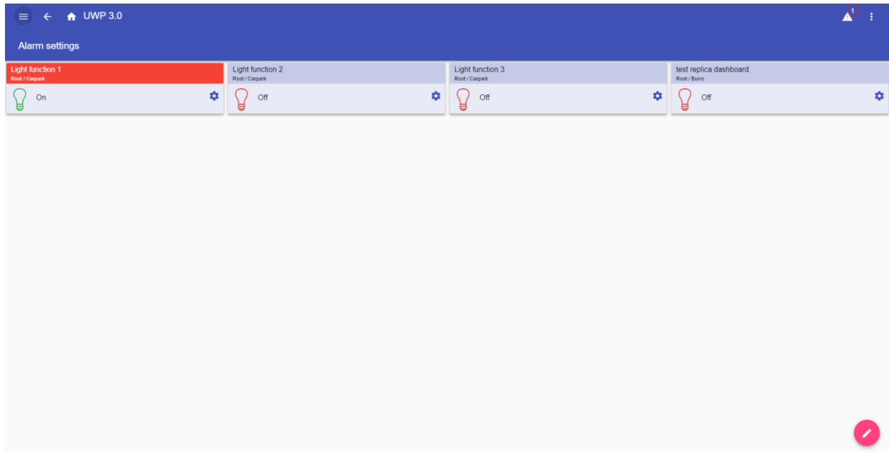
69. Alarmseite
