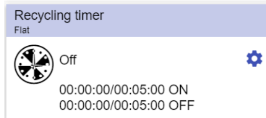
62. Recycling-Timer-Funktion
