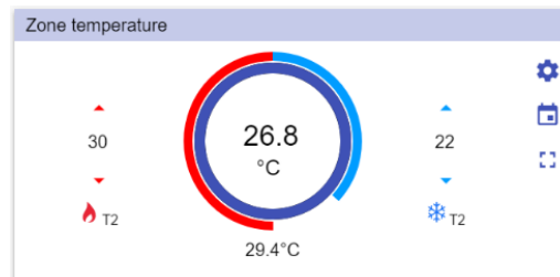
49. Zonentemperaturfunktion
