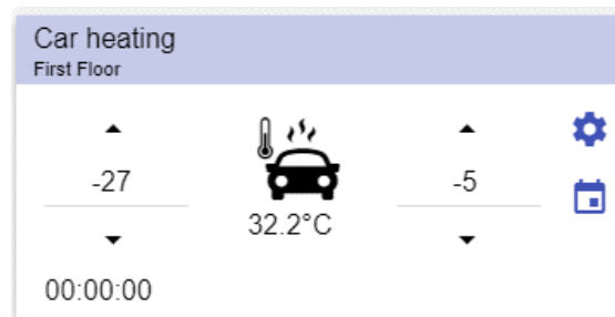
57. Autoheizfunktion
