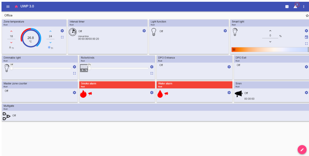
31. Widget Dashboard
