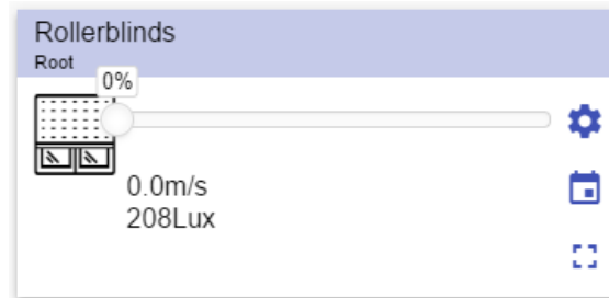
52. Rolladenfunktion
