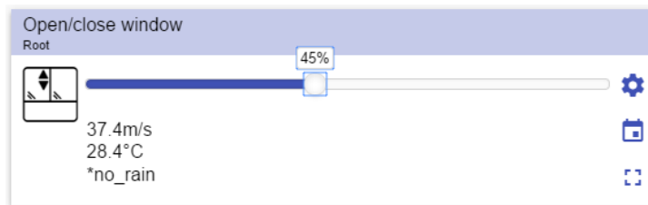
54. Windsteuerungsfunktion
