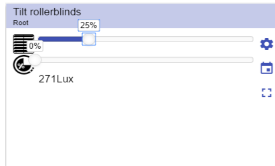
53. Rolladen-Neigungsfunktion
