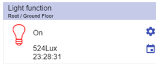
45. Lichtfunktion
