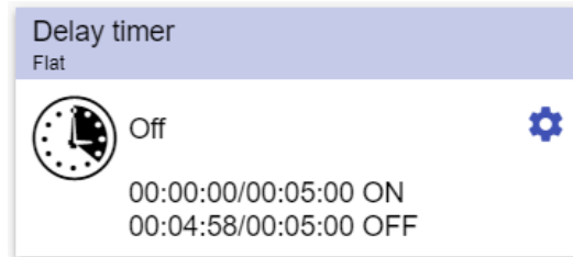
61. Timerverzögerungs-Funktion
