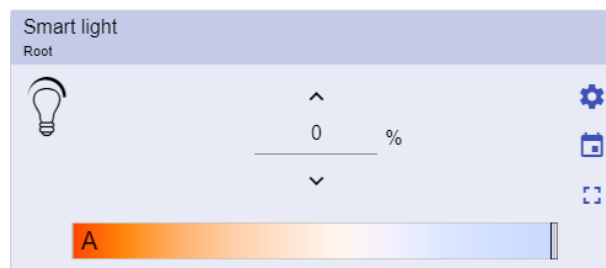
48. Funktion Smart-Licht
