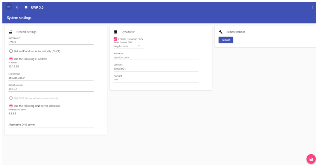
25. Systemeinstellungen
