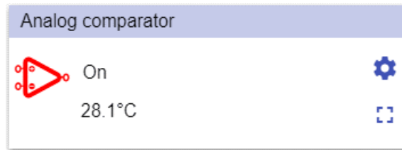
63. Analogvergleichsfunktion
