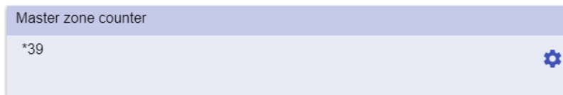
65. Master-Zonenzähler
