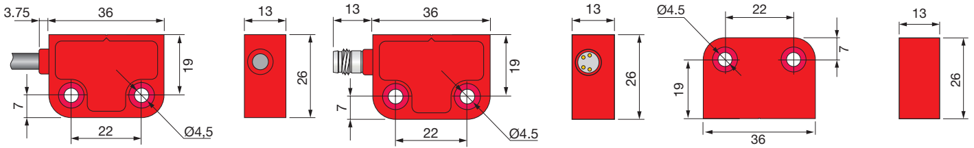
图 1 - 尺寸
