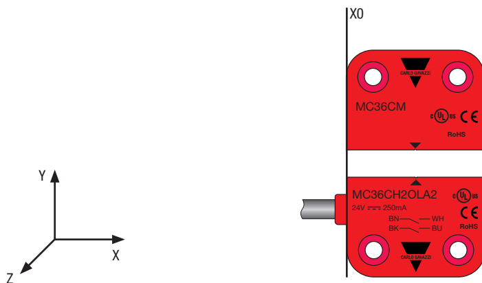
图 2 - 传感器的工作和对准方向
