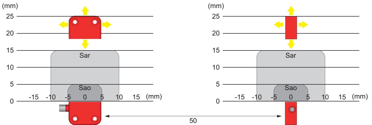
图 3 - 距离
