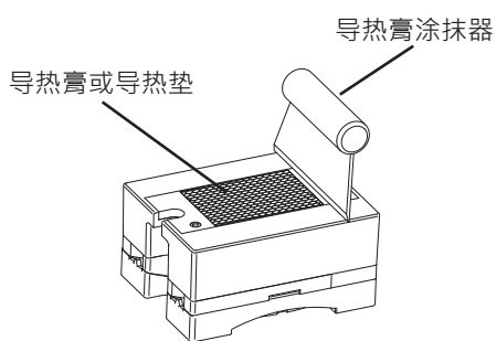
Fig. 11 应先在 SSR 的底座上均匀涂抹一层薄薄的导热硅膏，再将其安装到散热器上。也可以使用散热垫来代替。热界面材料会影响热性能。请确保散热器尺寸适当。
