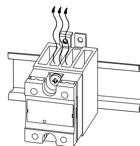
Fig. 13 安装散热器，使散热片处于垂直方向，以确保穿过散热器的最佳气流。
