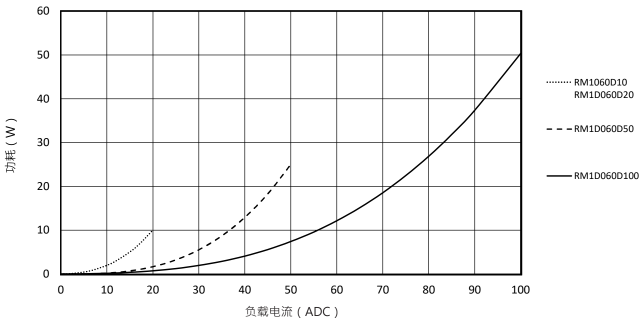
Fig. 7 输出功率损耗图
