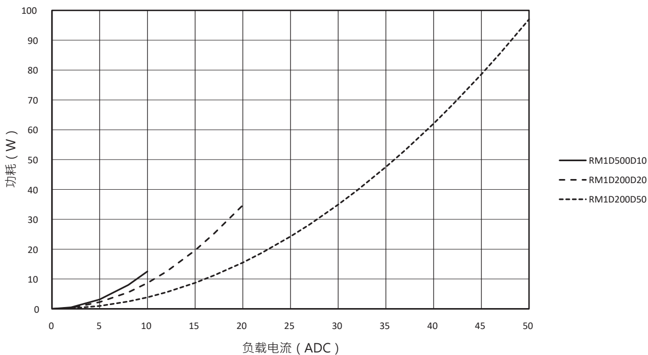
Fig. 8 输出功率损耗图
