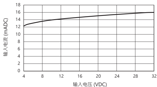
Fig. 3 输入电压与输入电流的关系曲线
